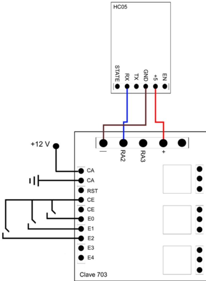
TRANSMISOR BT-TR3
